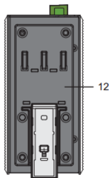
Вид сзади
