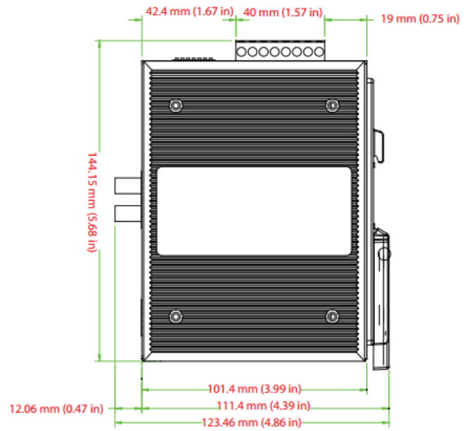
Вид сбоку (модель LV)
