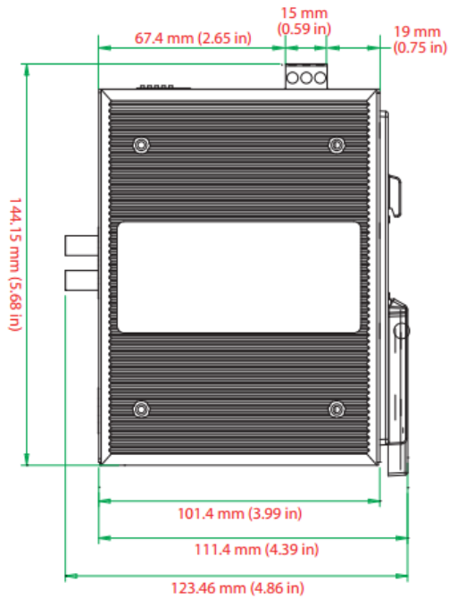
Вид сбоку (модель HV)
