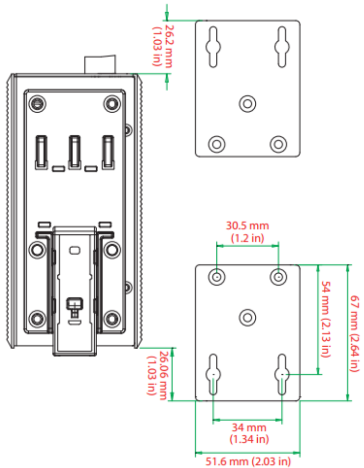
Вид сзади
