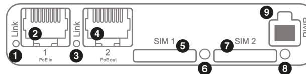
Изображение 2. Вид спереди R11-A.Wn
